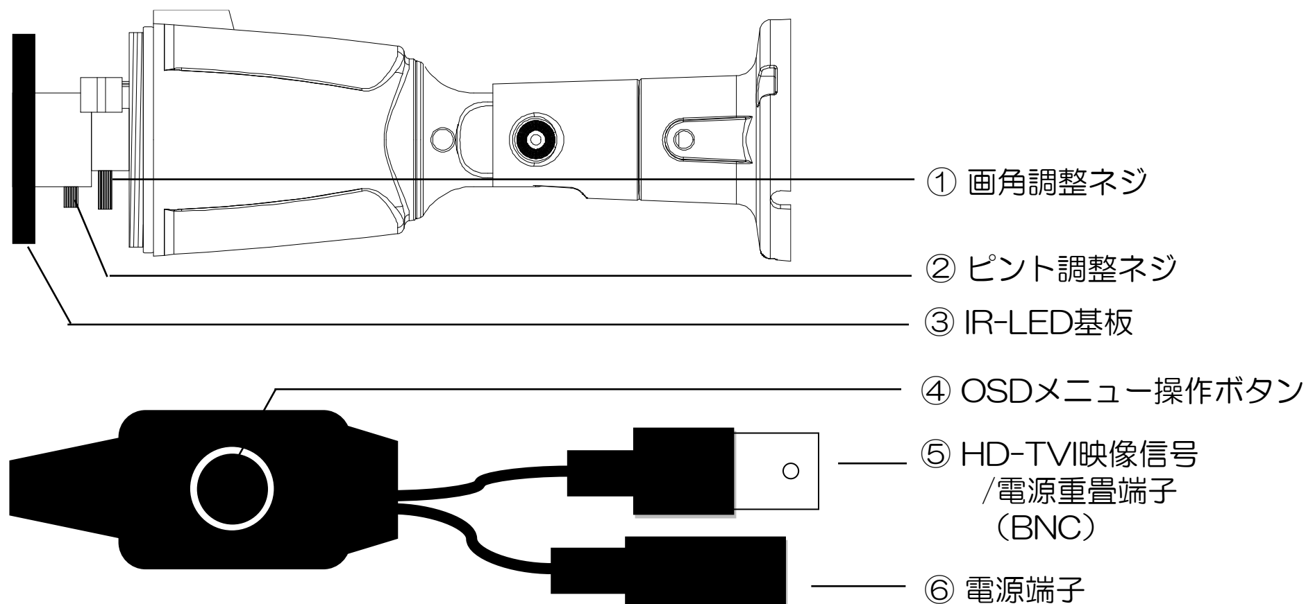
フロントカバーを外した図
