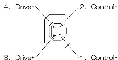
DC オートアイリスコネクタのピン配置
