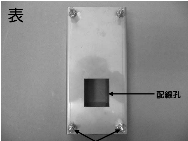
ドームハウジングブラケット取付ボルト(4箇所) ナット、スプリングワッシャー、ワッシャー
