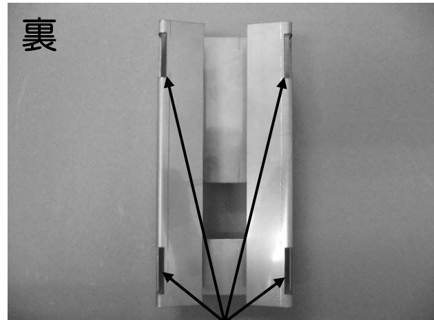
ポールバンド取付口 (4箇所) 取付口寸法: 33x9 (mm)
